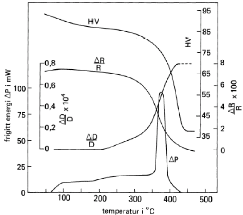
Figur 8.6 Frigitt energi \Delta P under avspenning og rekrySTALLISASJON av kalddeformert teknisk kobber. HV = Hardhet Vickers \Delta D/D = forandring i relativ tetthet (densitet) \Delta R/R = forandring i relativ resistivitet (elektrisk motstandsevne).
