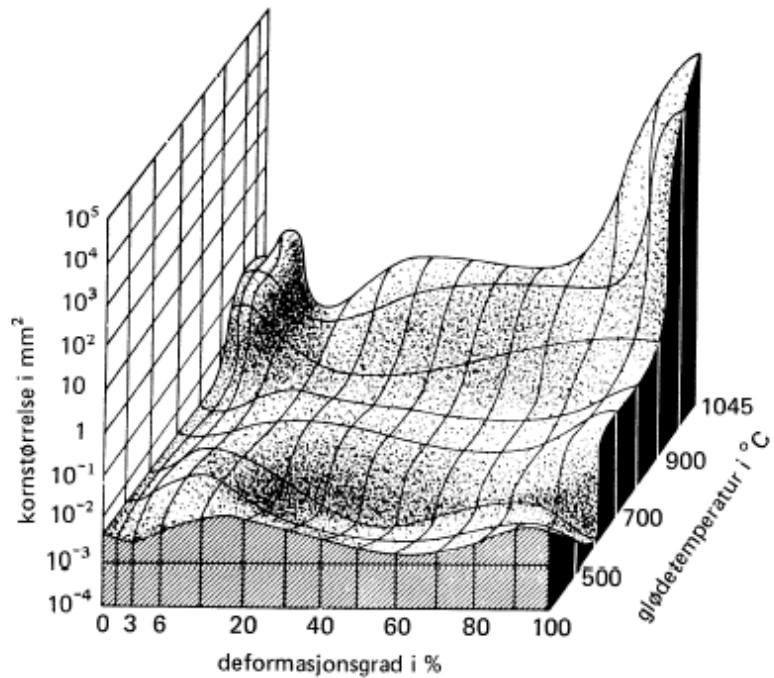
Figur 8.12 Kornstørrelse ved rekrySTALLISASJON av kobber Cu avhengig av deformasjons-grad og glødetemperatur. Glødetid er 30minutter.
