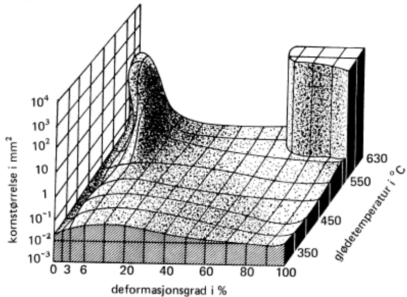
Figur 8.13 Kornstørrelse ved rekrySTALLISASJON av ren aluminium Al avhengig av deformasjonsgrad og glødetemperatur. Glødetid er 30minutter.
