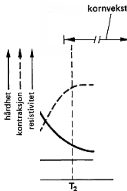
Figur 8.11 Kornvekst.
