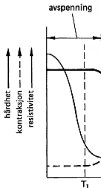
Figur 8.5 Avspenning.
