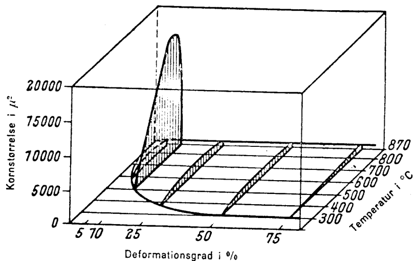
Figur 8.14 Kornstørrelse ved rekrySTALLISASJON av bløtt stål med ca. 0,1 % karbon avhengig av deformasjons- grad og glødetemperatur. Glødetid er 30minutter.
